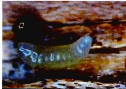
Рис. 7. Личинка Dinotiscus eupterus , питающаяся личинкой уссурийского полиграфа
