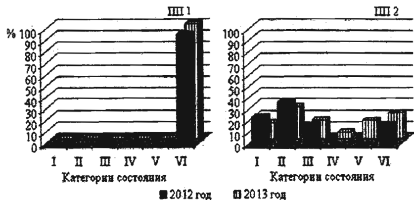
Рис. 16. Распределение деревьев пихты сибирской по категориям состояния на пробных площадях в Ларинском ландшафтном заказнике (Томская область), поврежденном уссурийским полиграфом, рассчитанное по сумме площадей поперечного сечения стволов. Категории состояния деревьев: I – здоровые; II – ослабленные; III – сильно ослабленные; IV – усыхающие; V – свежий сухостой, VI – старый сухостой
