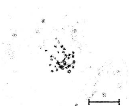
Рис. 2. Кариотип Armeniaca sibirica ( 2n=32 ). Масштабная линейка 10 мкм.
