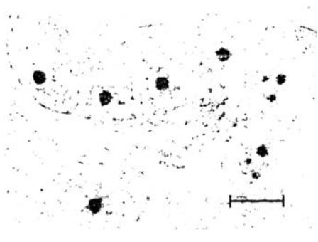
Рис. 3. Разное число ядрышек в интерфазных ядрах Armeniaca sibirica . Масштабная линейка 10 мкм.
