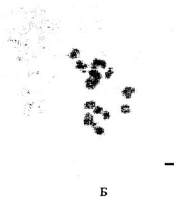
Рис. 1. Кариотип Armeniaca sibirica ( 2n=16 ) А. Об. 100\times , ок. 10\times . Масштабная линейка 10 мкм. Б. Масштабная линейка 1 мкм
