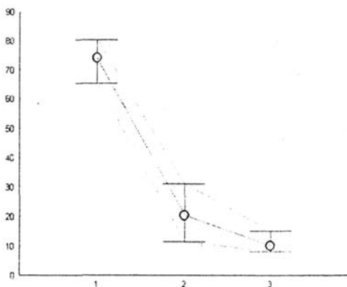
Рис. 4. Число ядрышек в интерфазных ядрах Armeniaca sibirica .
